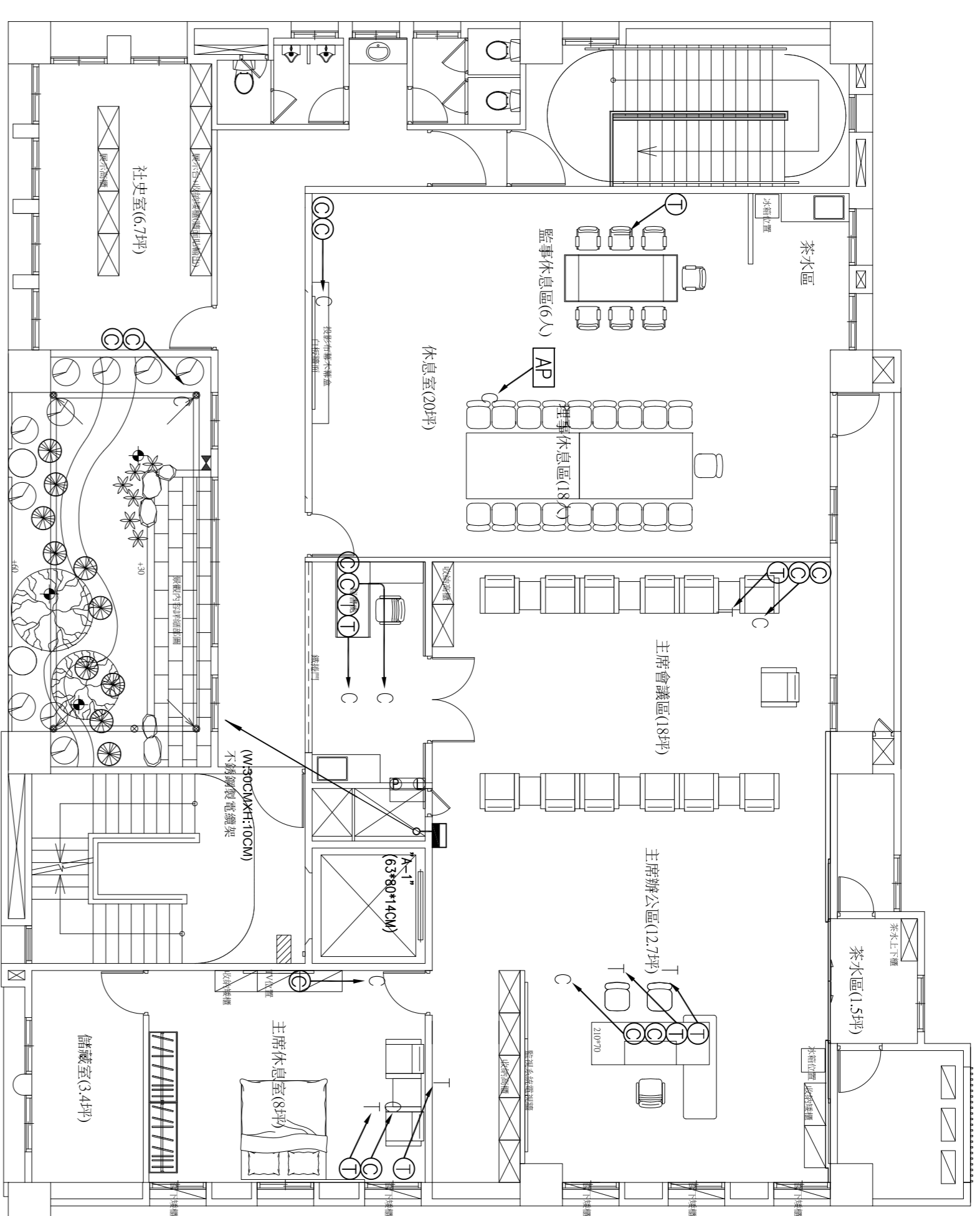
五層平面圖 S=1:100
